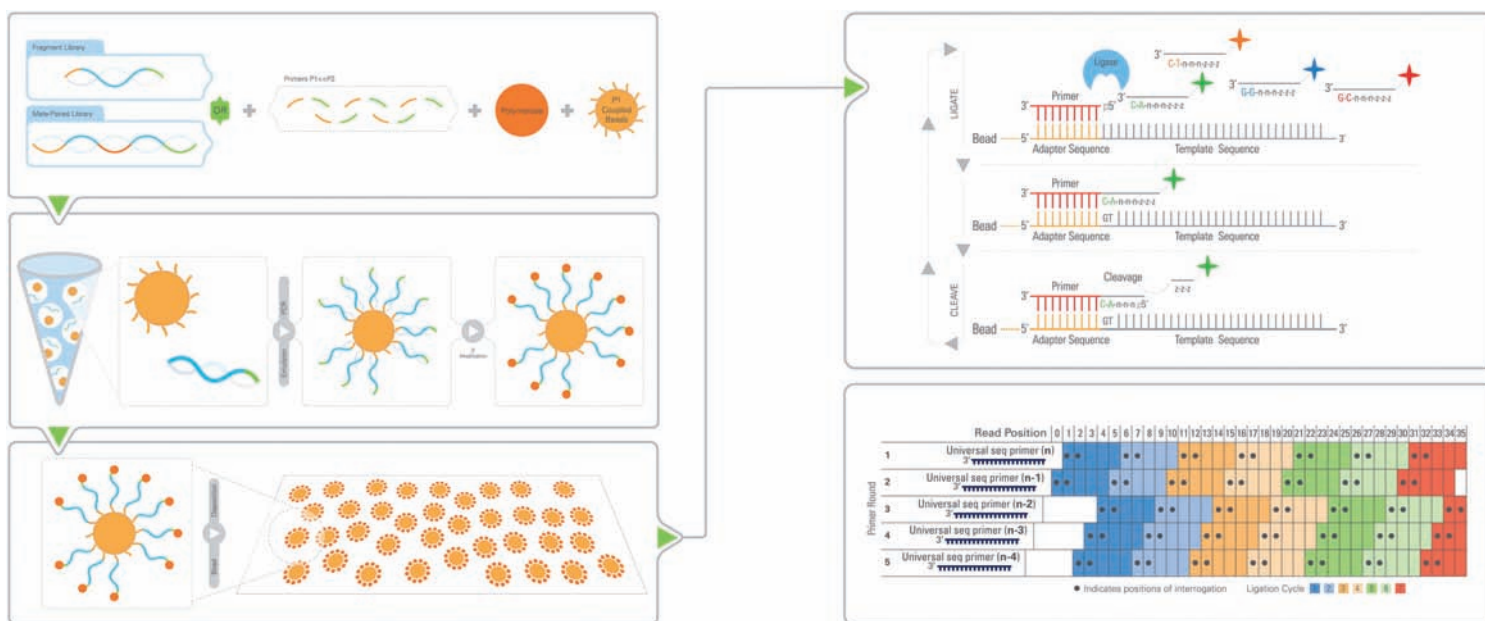
Método de “secuenciación por ligamiento” del sistema Applied Biosystems SOLiD™ 4
