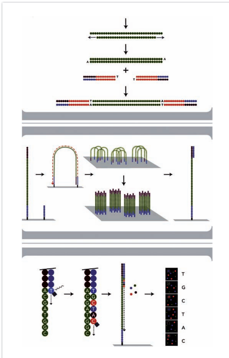
Fig. 2. ▲ Método de "secuenciación por síntesis" del sistema Genome Analyzer Iix de Illumina
